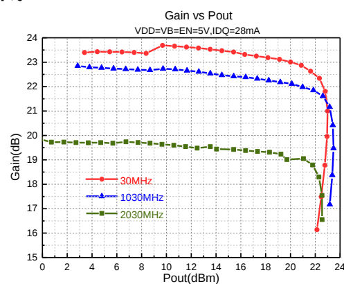
增益曲线
